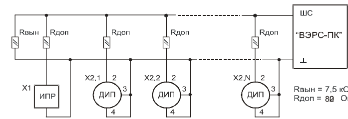
Рис.П3. Схемы включения ШС типа ШННС и ШПНС с несколькими дымовыми извещателями (типа ИП212) и сработкой по двум извещателям (с перезапросом).
