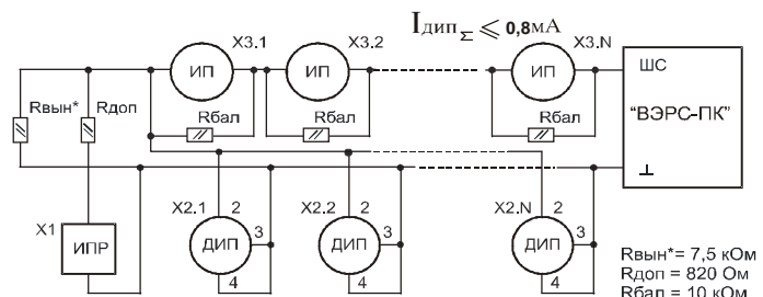
Рис.П5. Комбинированная схема включения ШС типа ШННС со сработкой по одному извещателю (с перезапросом).
